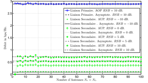
FIG. 3: Débit Asymptotique du système opportuniste avec AUP observée par simulation comme fonction du nombre d'antennes quand N_r = N_t à différents niveaux de RSB. RSB = \frac{p_{\max}}{\sigma^2} . Les lignes noirs sont des asymptotes déterminées par le Th. 6. Les asymptotes du système primaire sont données par [10].
